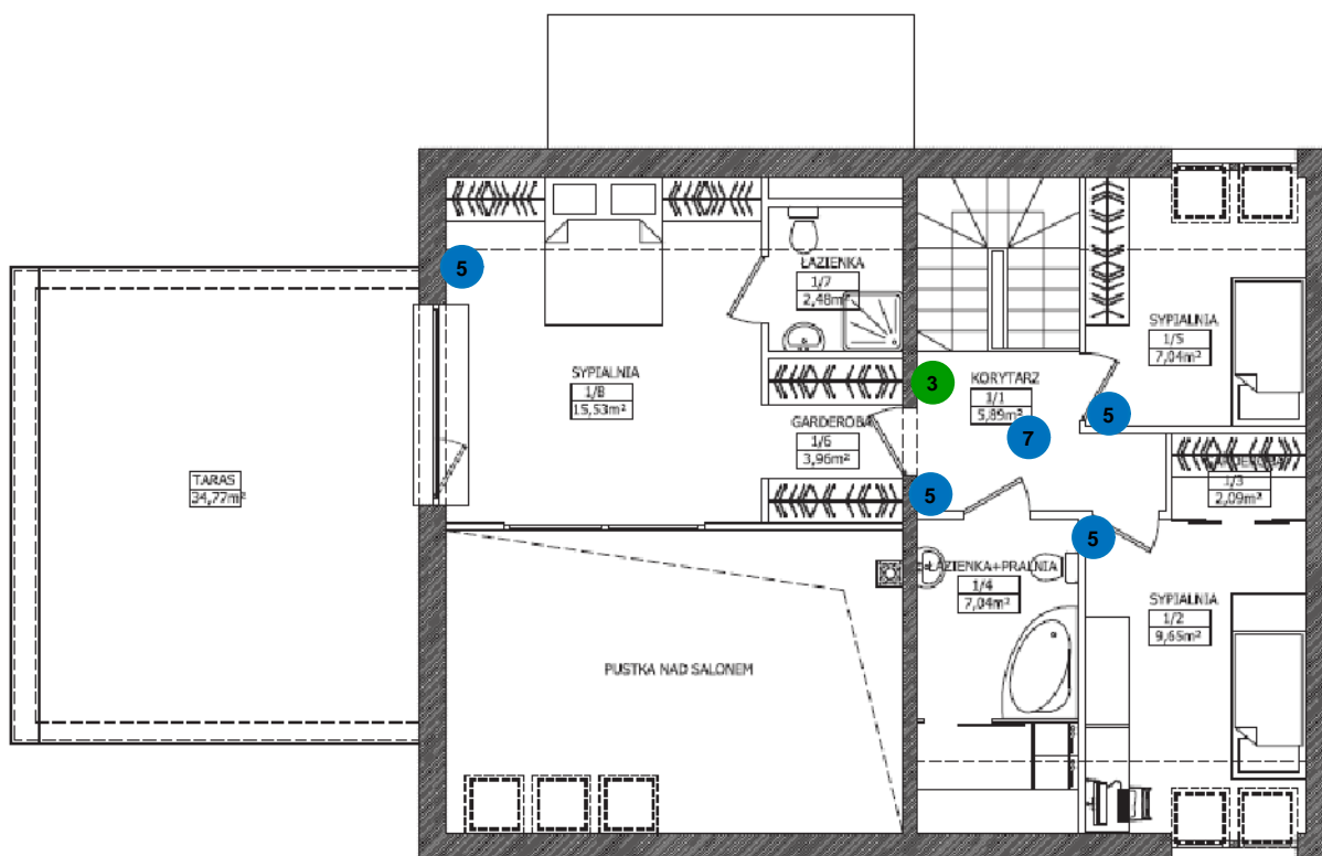
PRZYKŁADOWY RZUT PIĘTRA
